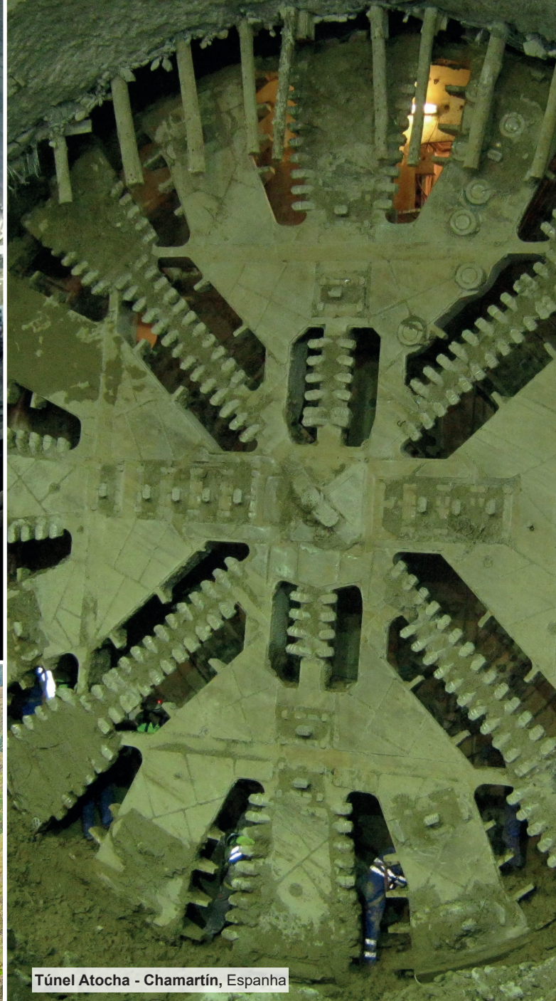
Túnel Guillermo Gaviria Echeverri, Colombia
